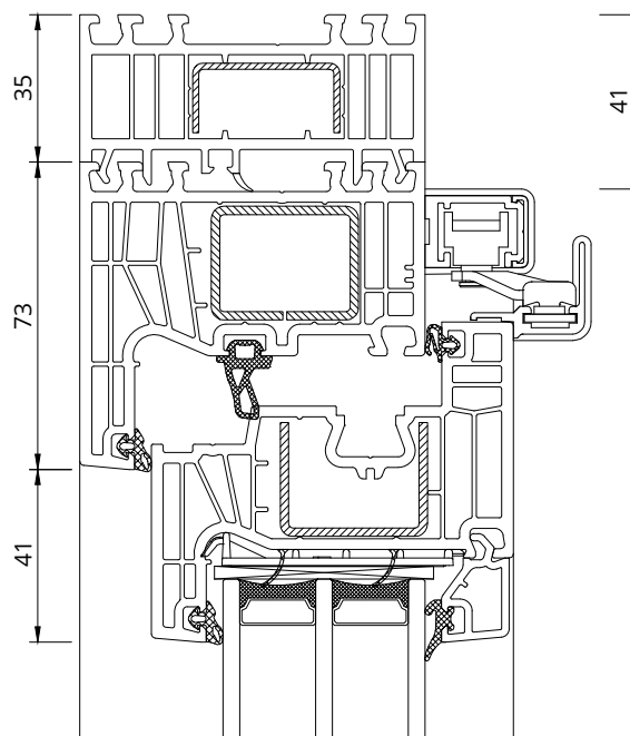
A - A
