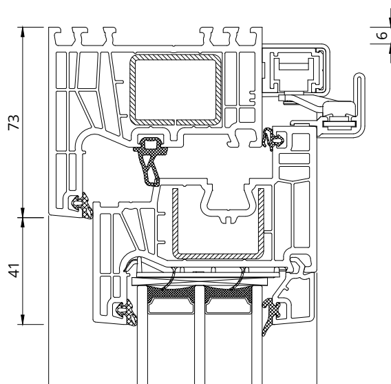
A - A
