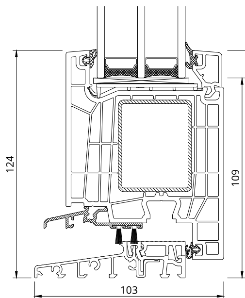
Combi 20mm + 80033 + 50930A
