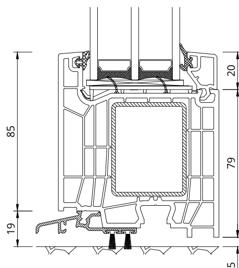
80033 + 50930A bez progu without thereschold Ohne Schwelle senza soglia
