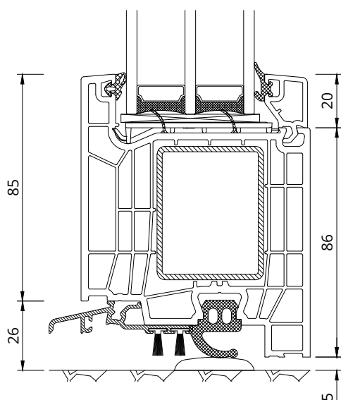
80033 + 50930A niski próg - łódeczkowy thereshold 5mm Schwelle 5mm soglia bassa - a sfera
