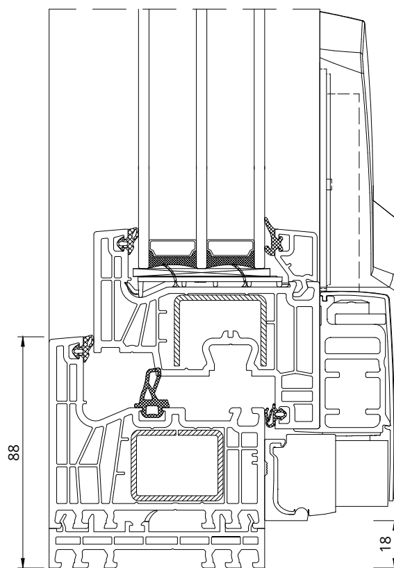
B - B
