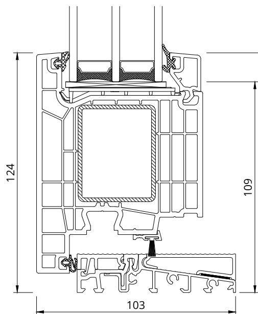
Combi 20mm + 80034 + 50930A
