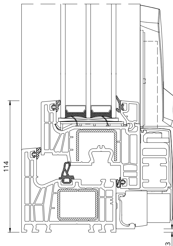
B - B
